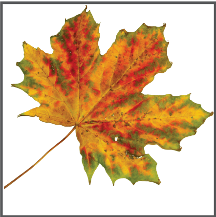
8. BLOAT TOOL
