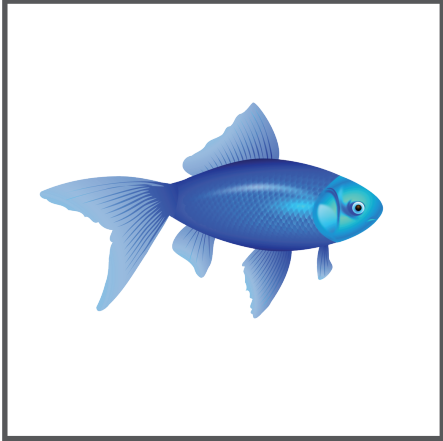
4. REFLECT TOOL
